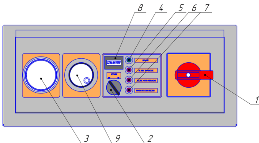
Рис. 3. Панель управления
