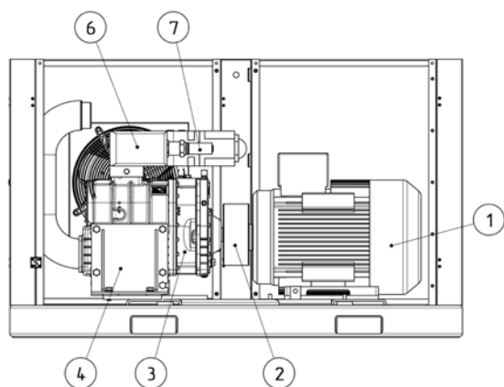
Рис. 2. Общий вид установки
